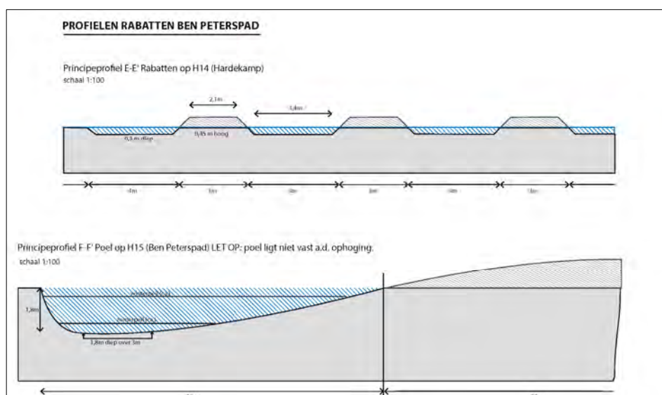
Figuur 2-3: Profielen locatie Hardekamp, rabatten bij het Ben Peterspad (22-06-2020)
