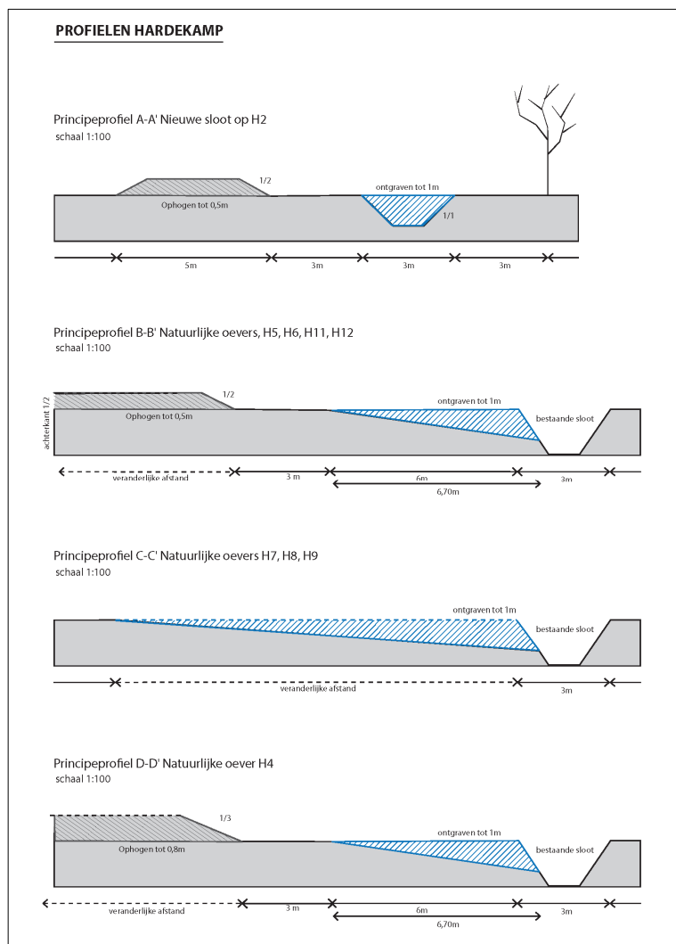
Figuur 2-2: Profielen grondverzet locatie Hardekamp (22-06-2020)
