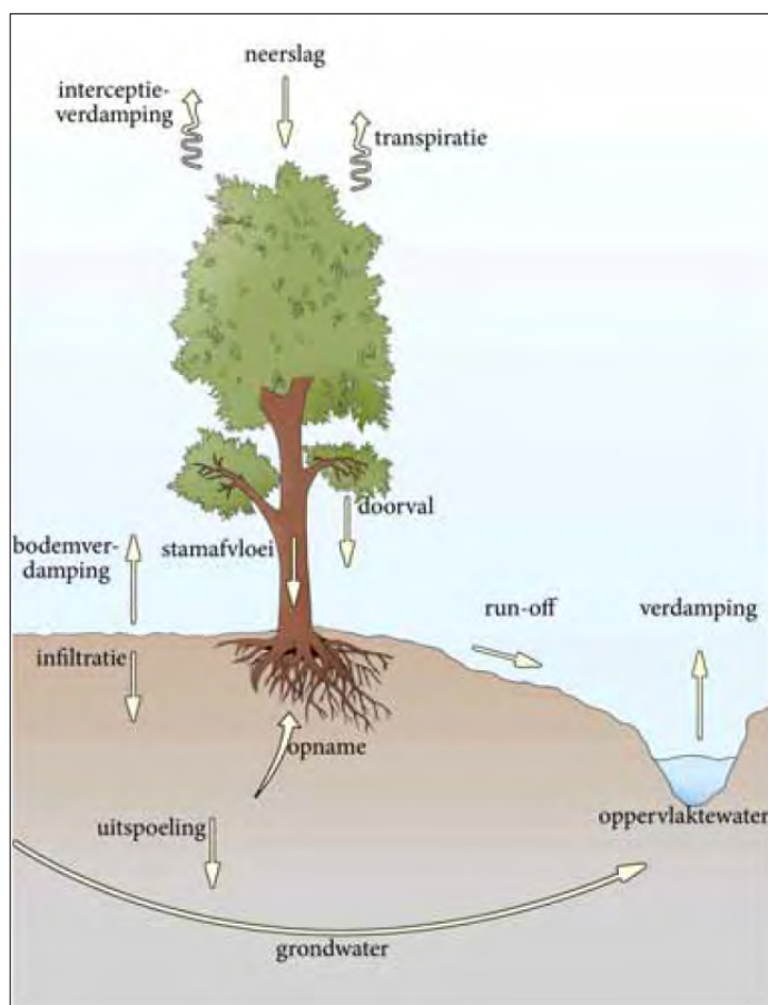
Figuur 2-1 Schematische waterbalans van een bosesysteem. Uit den Ouden (2011). De neerslag wordt voor een deel via verdamping (transpiratie en interceptie) teruggeven aan de atmosfeer en voor een deel bereikt deze de grond, waar hij dan wel oppervlakkig afstroomt richting het oppervlaktewater, ofwel infiltreert richting het grondwater.
