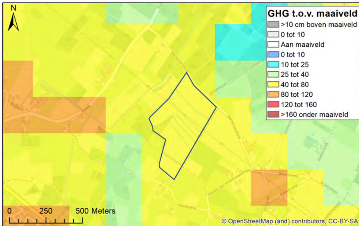
Figuur 3-3: Berekende GHG uit het Brabant-model (RHDHV, 2019)
