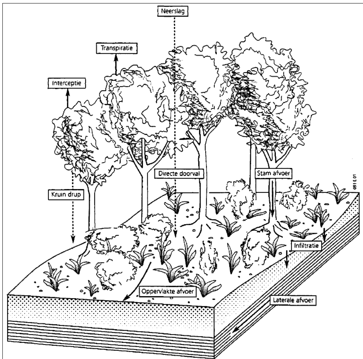
Figuur 2-3 Schematische waterbalans van een bosecosysteem. Uit (Dolman & Moors 1994). De neerslag wordt voor een deel via verdamping (transpiratie en interceptie) teruggeven aan de atmosfeer en voor een deel bereikt deze de grond, waar hij dan wel oppervlakkig afstroomt richting het oppervlaktewater, ofwel infiltreert richting het grondwater.
