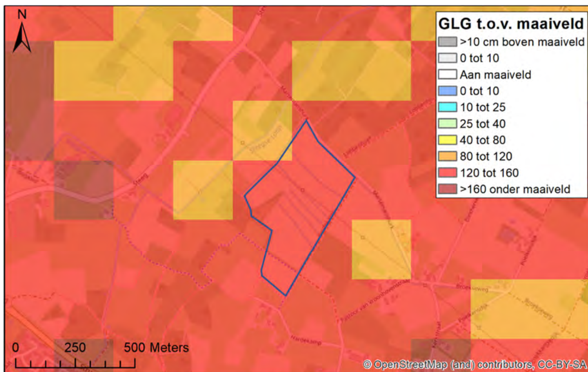
Figuur 3-4: Berekende GLG uit het Brabant-model (RHDHV, 2019)
